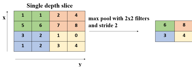
Fig. 6. Max Pooling
