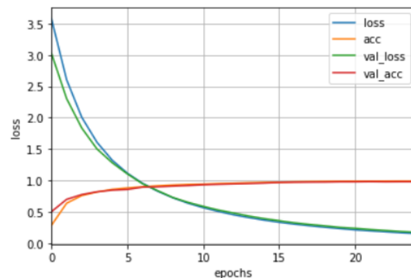
Fig. 9. VGG16
